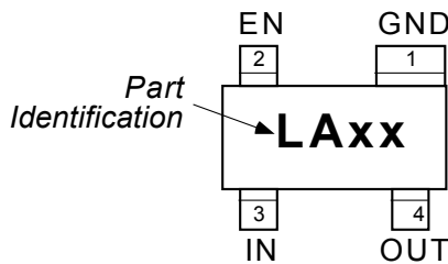
SOT-143 (M4)
