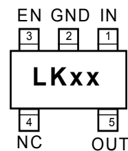
SOT-23-5 (M5)
